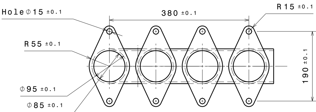
Top view Scale: 1:6
