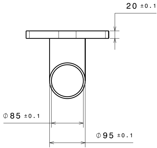
Right view Scale: 1:6
